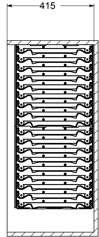
DOORSNEDE B-B
