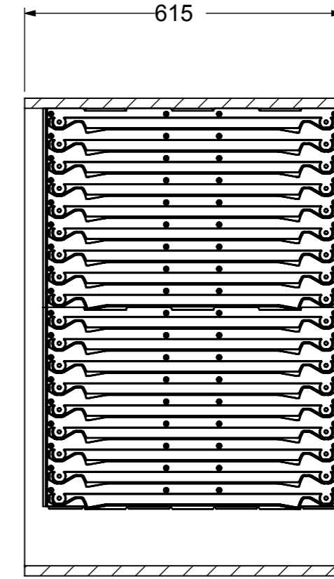
DOORSNEDE D-D
